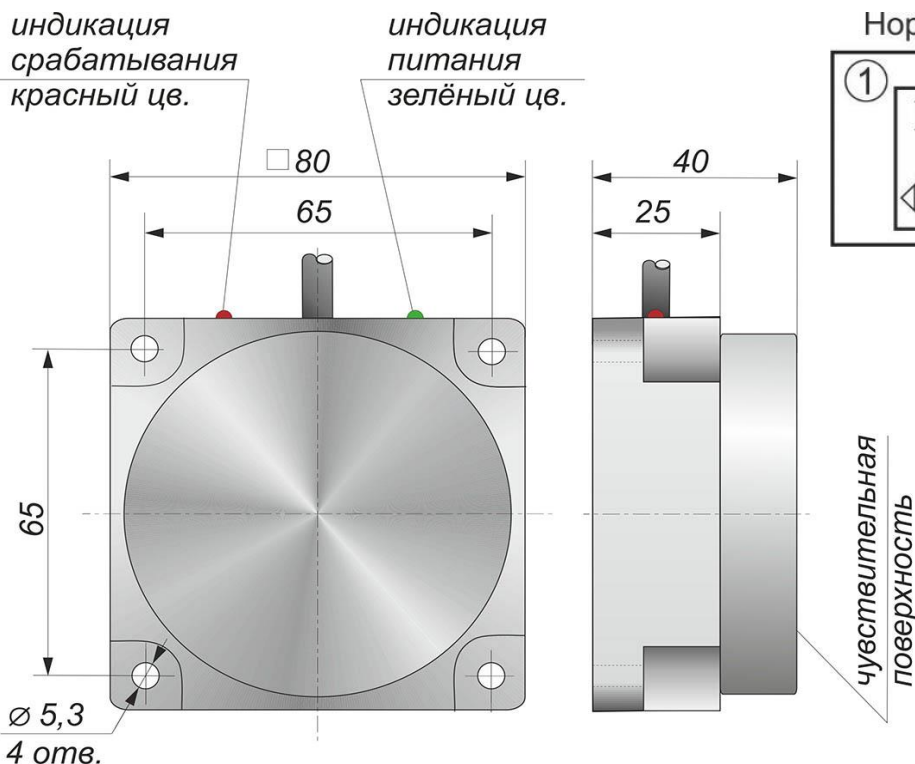
Габаритный чертеж
