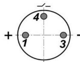
Цоколевка разъема
