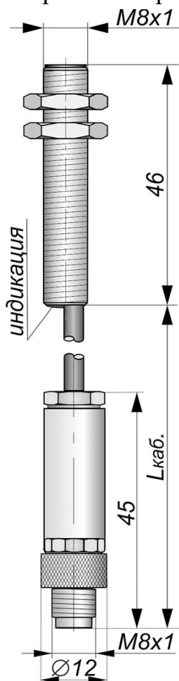
Габаритный чертеж
