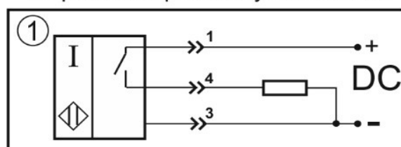
Нормально-разомкнутый контакт
