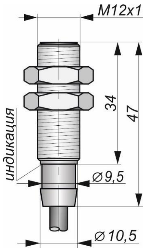
Габаритный чертеж
