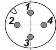
Цоколевка разъема
