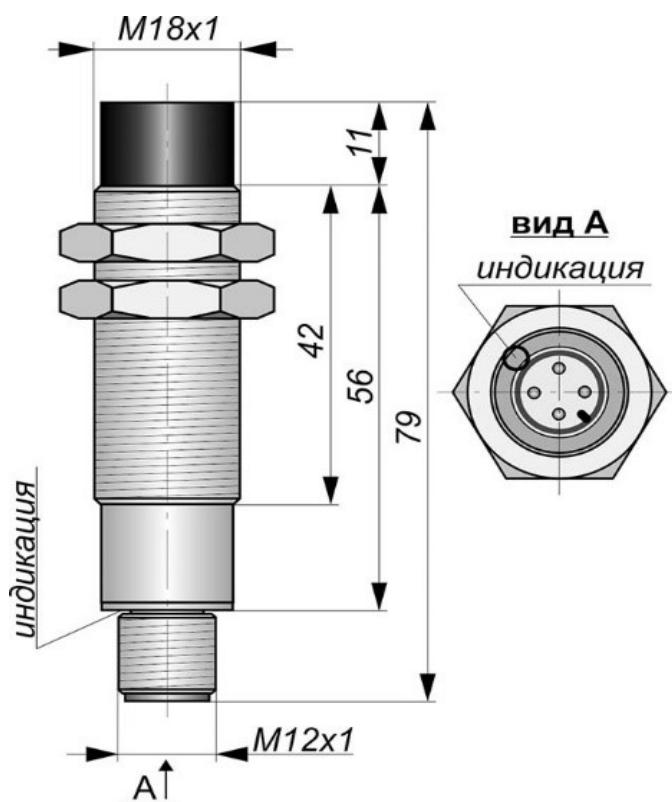
Габаритный чертеж
