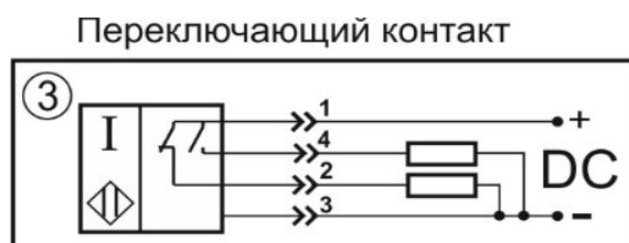
Цоколевка разъема
