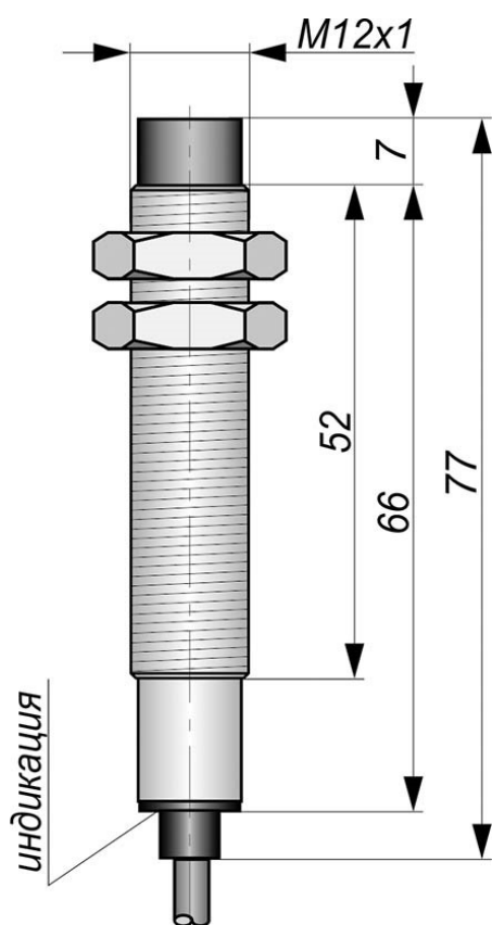
Габаритный чертеж
