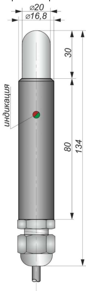
Габаритный чертеж
