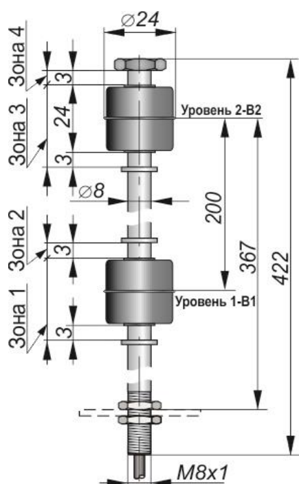
Габаритный чертеж
