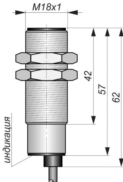
Габаритный чертеж
