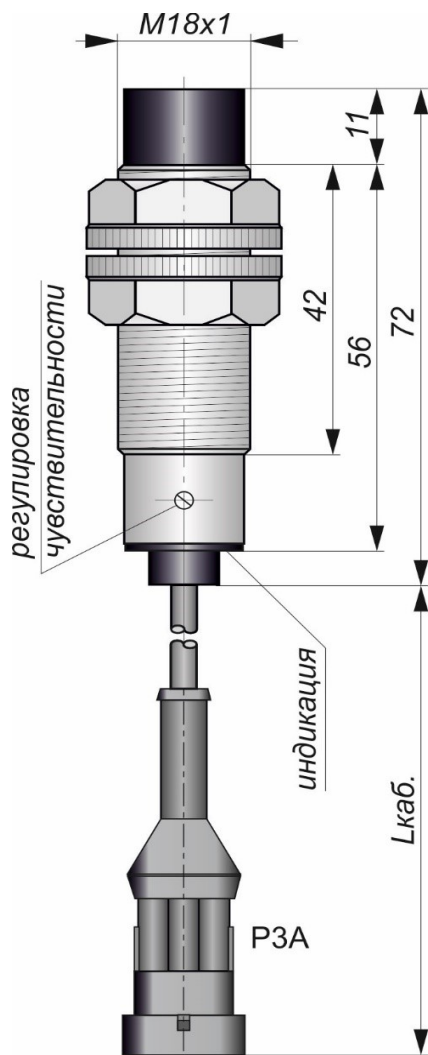
Габаритный чертеж
