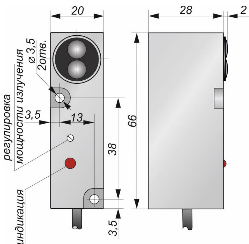
Габаритный чертеж
