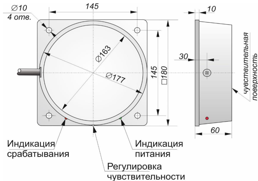
Габаритный чертеж
