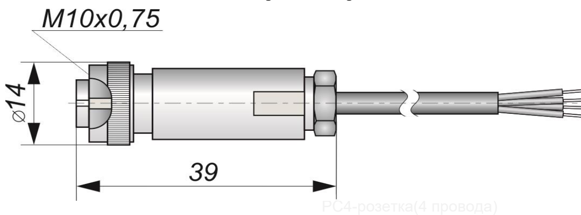
Габаритный чертеж
