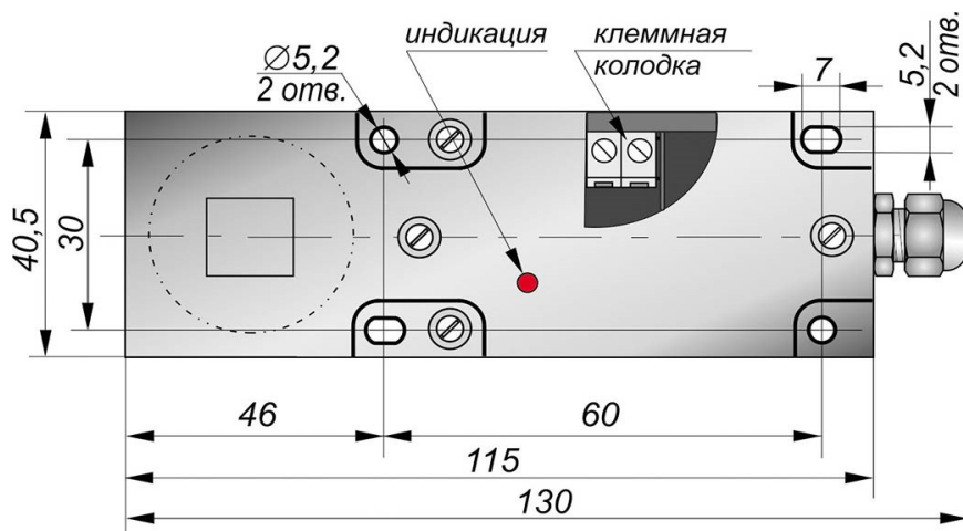
Вид со стороны чувствительного элемента
