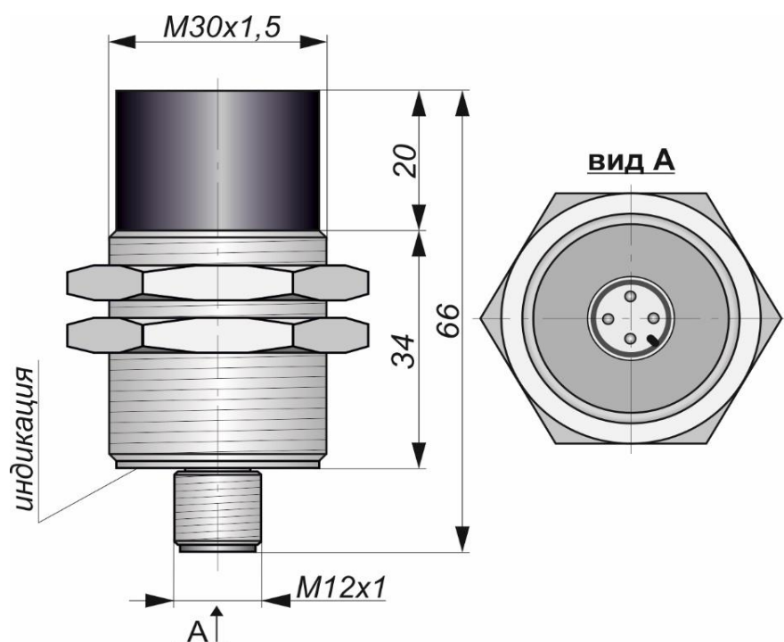
Габаритный чертеж
