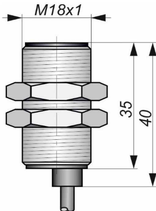
Габаритный чертеж
