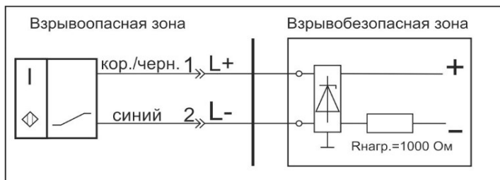
Схема соединения
