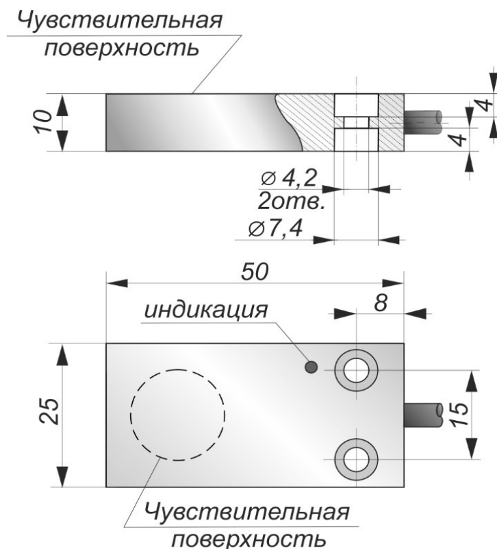
Габаритный чертеж
