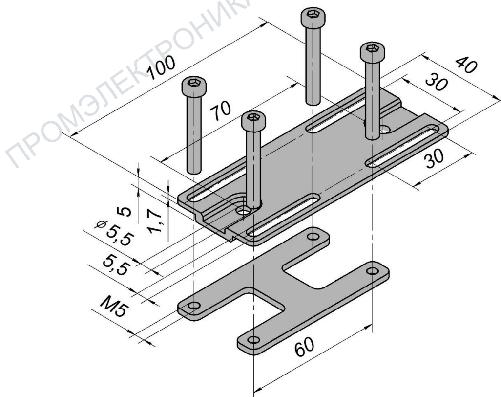
Габаритный чертеж
