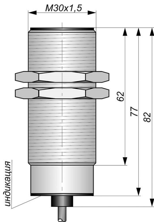
Габаритный чертеж
