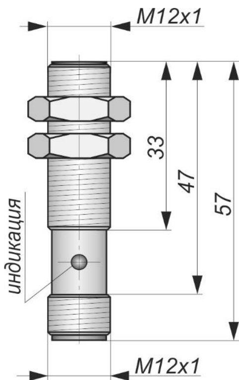
Габаритный чертеж
