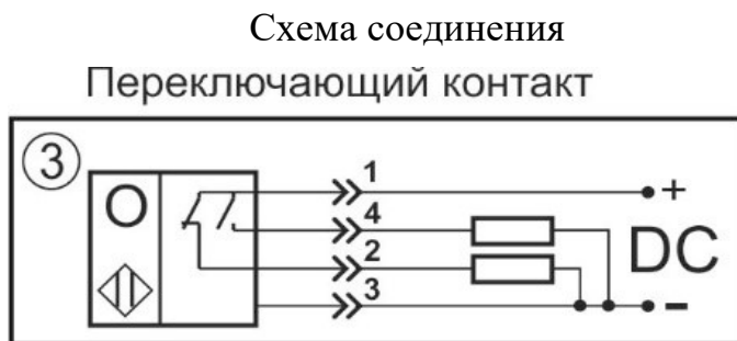
Цоколевка разъема
