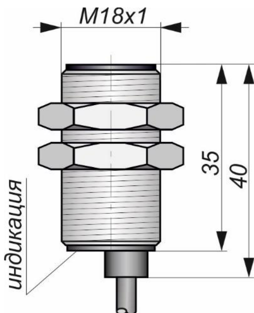
Габаритный чертеж
