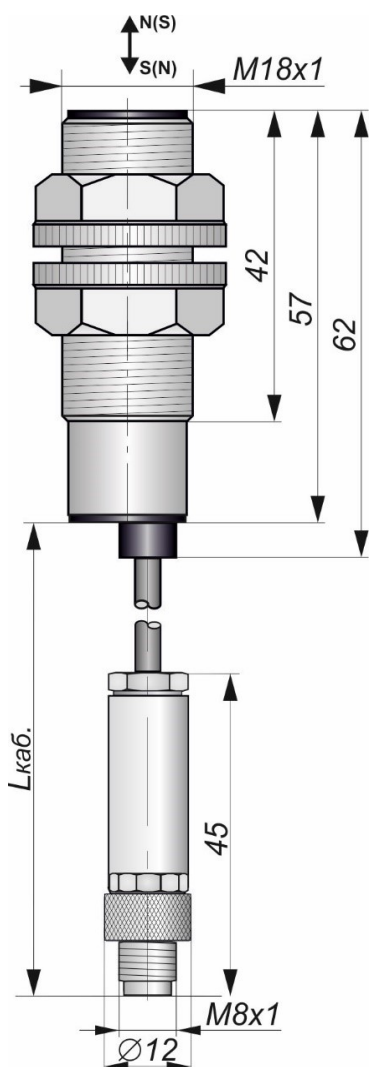
Габаритный чертеж
