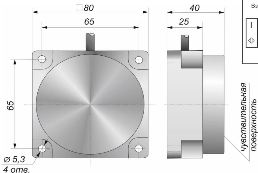
Габаритный чертеж
