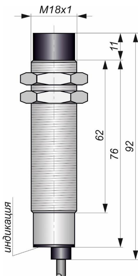
Габаритный чертеж
