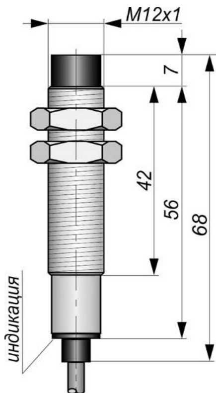
Габаритный чертеж
