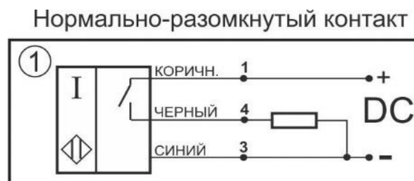
Схема соединения
