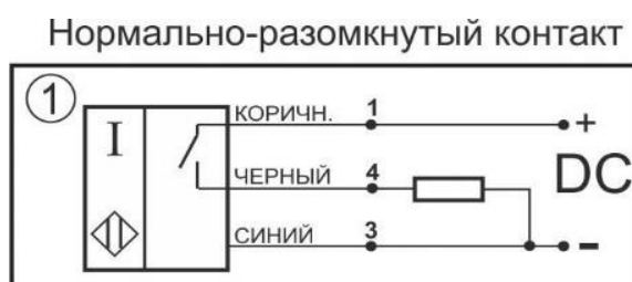
Схема соединения
