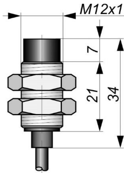
Габаритный чертеж
