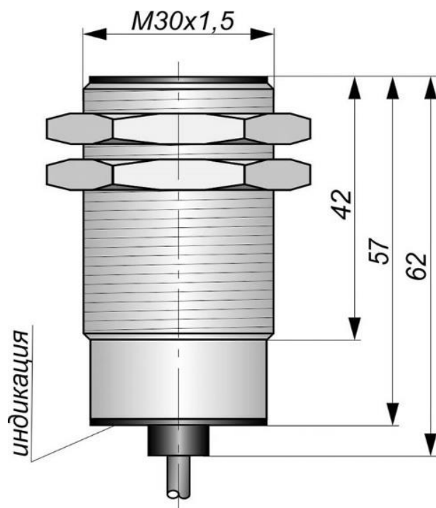
Габаритный чертеж
