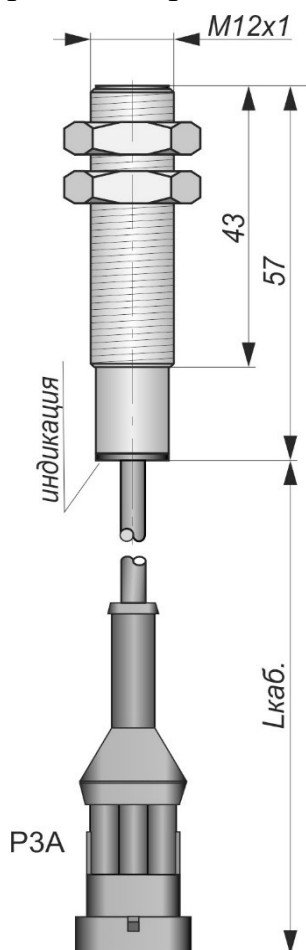
Габаритный чертеж
