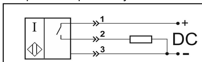
Нормально-разомкнутый контакт
