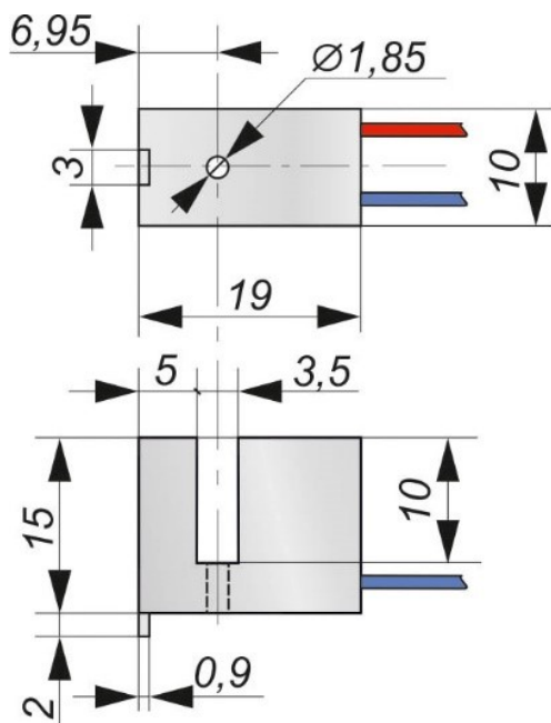
Габаритный чертеж
