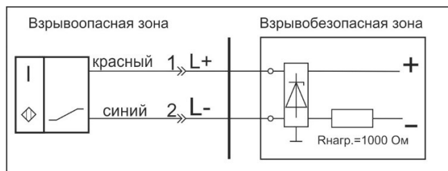
Схема соединения
