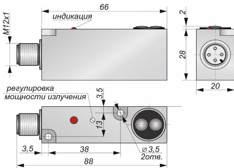
Габаритный чертеж
