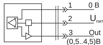
Схема присоединения
