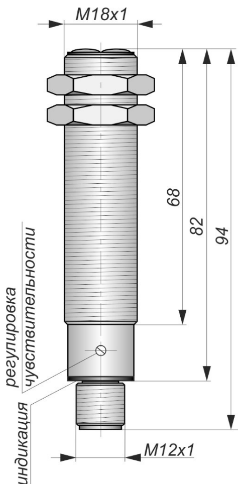
Габаритный чертеж
