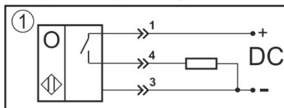
Цоколевка разъема
