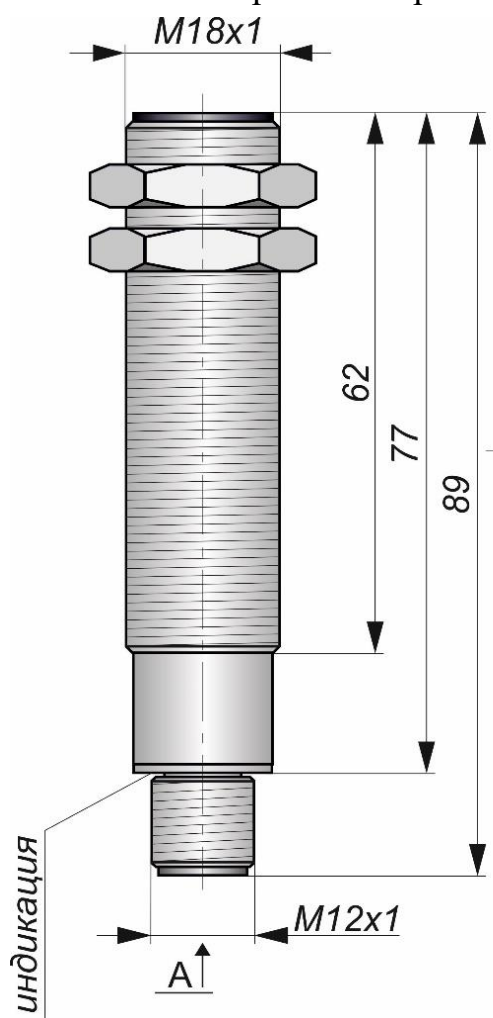
Габаритный чертеж
