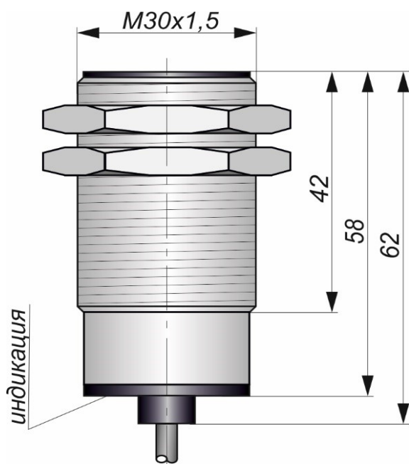
Габаритный чертеж
