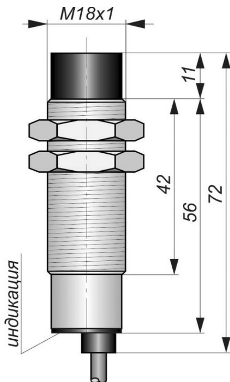
Габаритный чертеж
