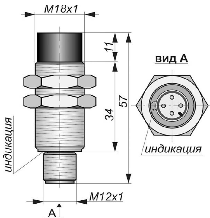
Габаритный чертеж
