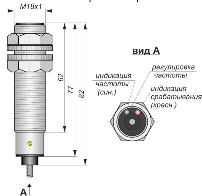
Габаритный чертеж
