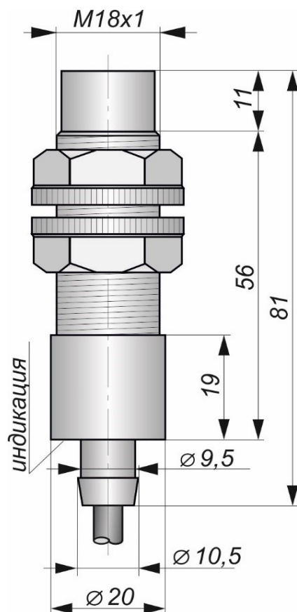
Габаритный чертеж
