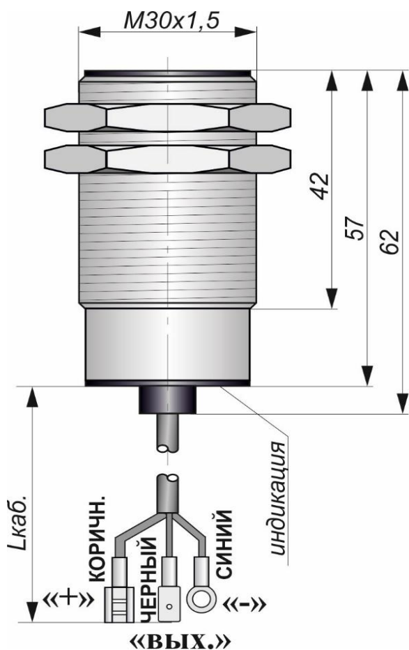
Габаритный чертеж
