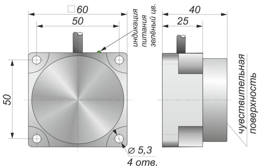
Габаритный чертеж
