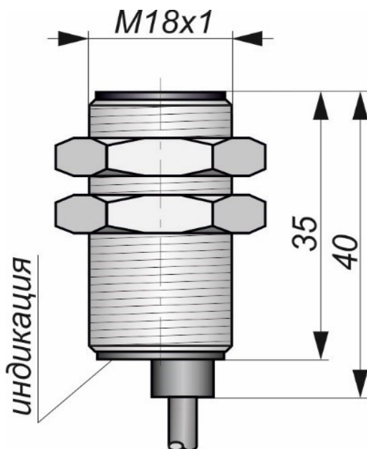
Габаритный чертеж
