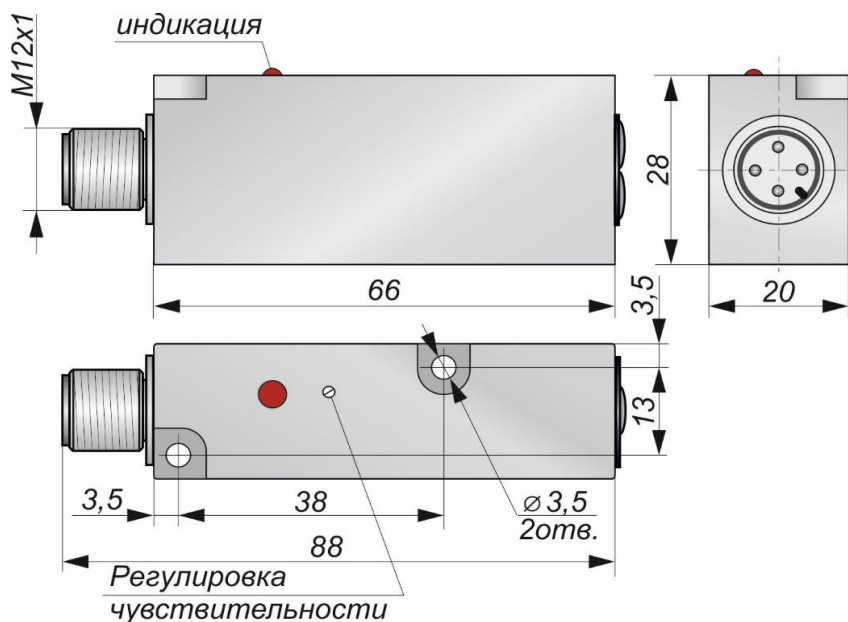
Габаритный чертеж
