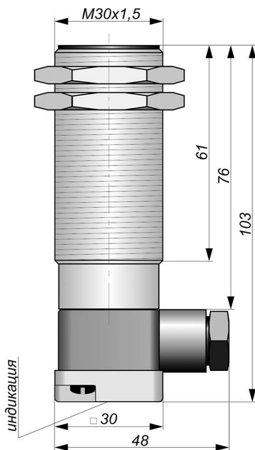
Габаритный чертеж
