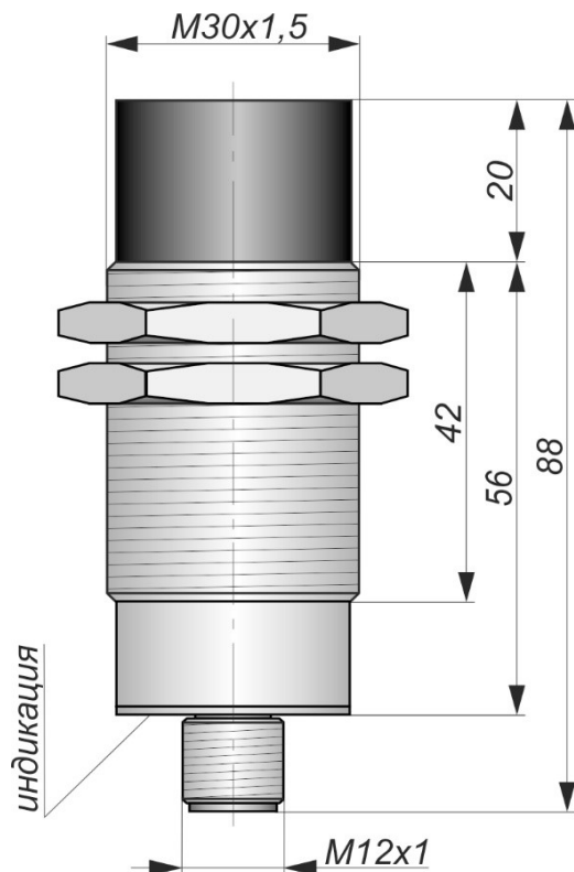
Габаритный чертеж
