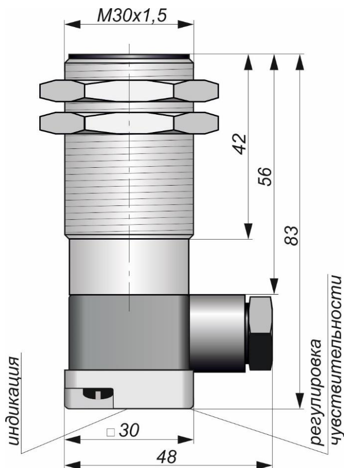
Габаритный чертеж
