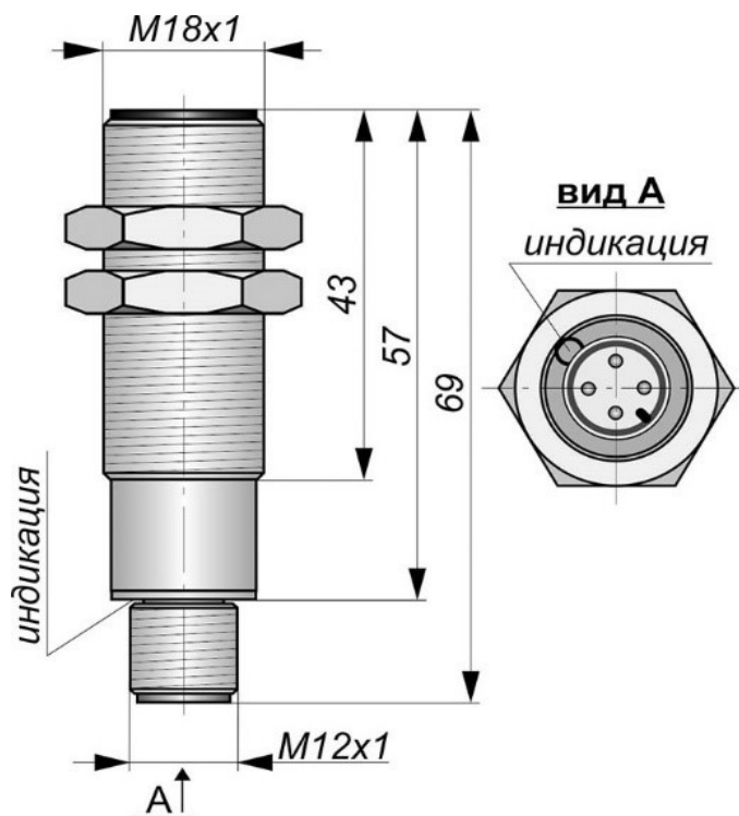
Габаритный чертеж
