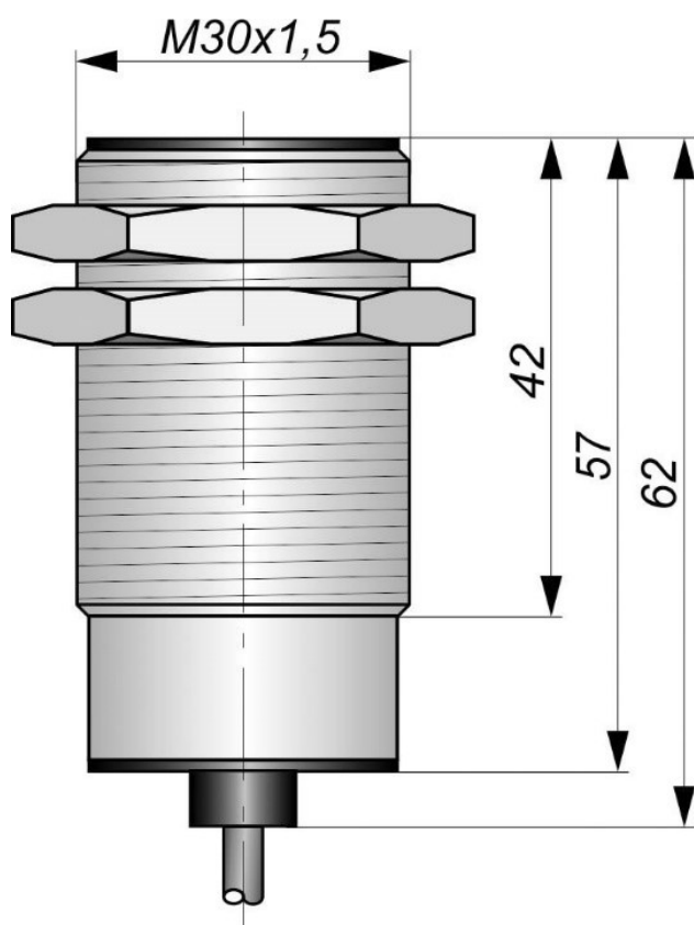
Габаритный чертеж
