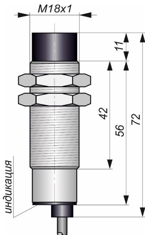
Габаритный чертеж
