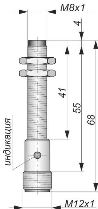
Габаритный чертеж
