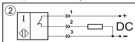
Нормально-замкнутый контакт
